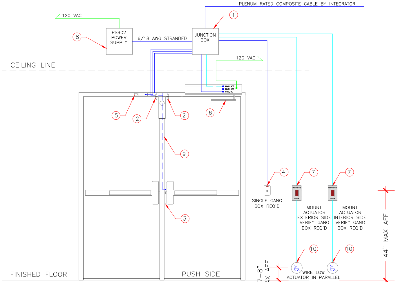
DOOR ELEVATION N.T.S.
